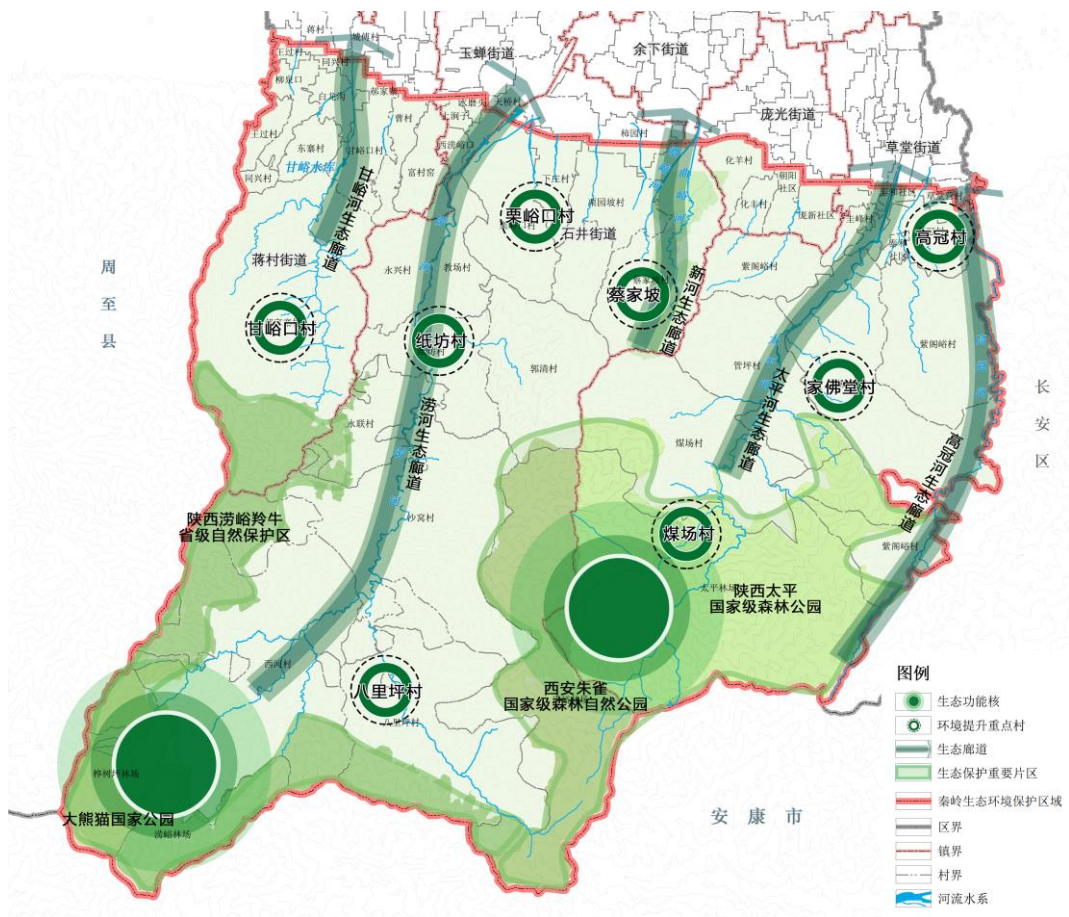
图 5-1 鄂邑区秦岭生态环境格局示意图
